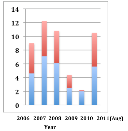
Replikin Count
