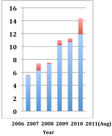
Replikin Count
